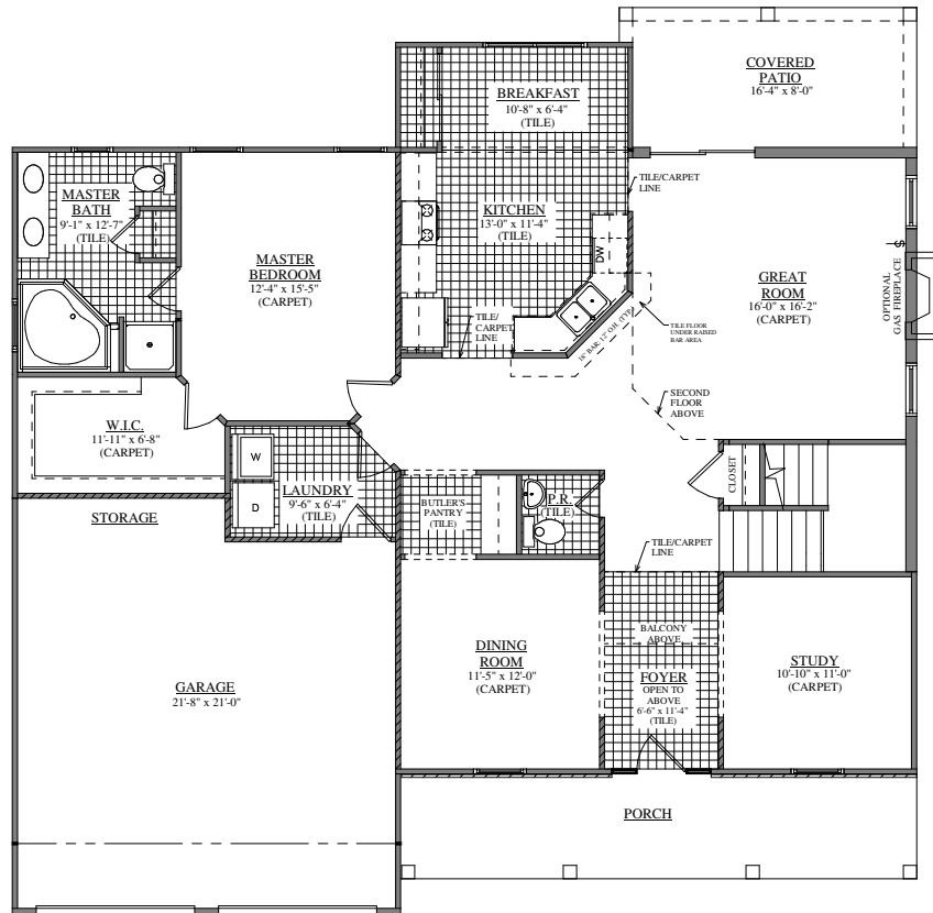
FIRST FLOOR PLAN FORINO - THE OKATIE (S.C. #4)
