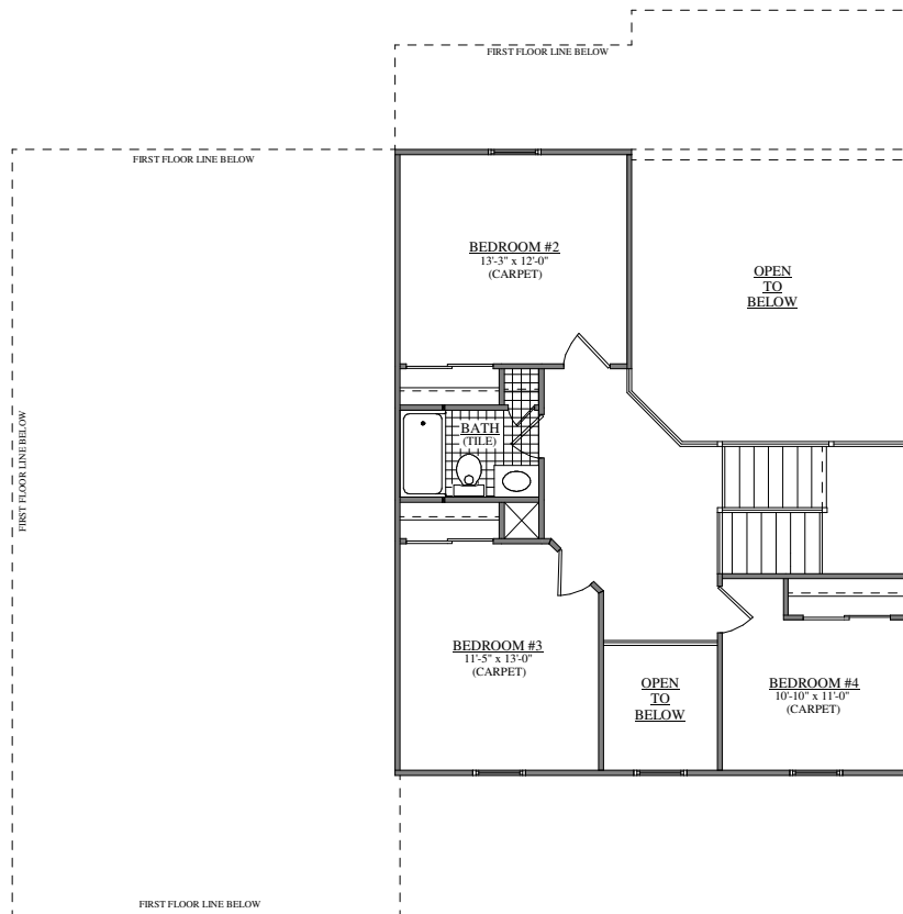
SECOND FLOOR PLAN FORINO - THE OKATIE (S.C. #4)
